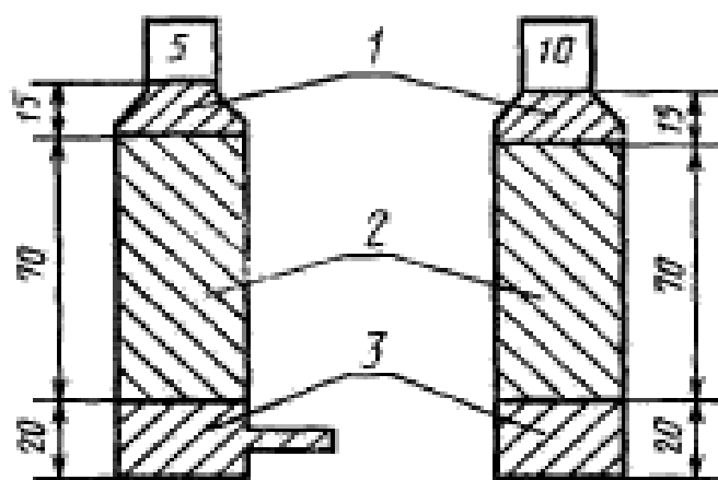
1 — стеклянная вата; 2 — абсорбент; 3 — стеклянная вата
