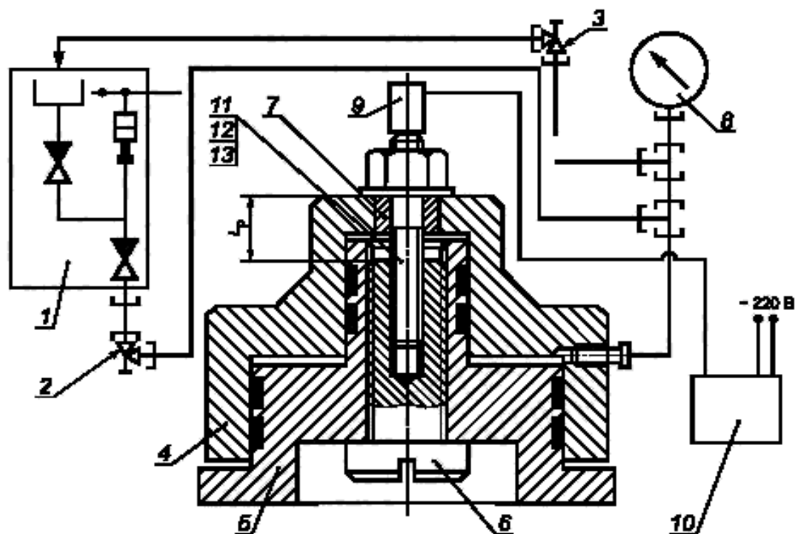
1 — гидравлический ручной насос; 2 — напорный вентиль; 3 — сливной вентиль; 4 — цилиндр; 5 — поршень; 6 — сменный винт; 7 — центрирующая втулка; 8 — манометр; 9 — ЗАП; 10 — прибор; 11 — шпилька; 12 — гайка; 13 — шайба
