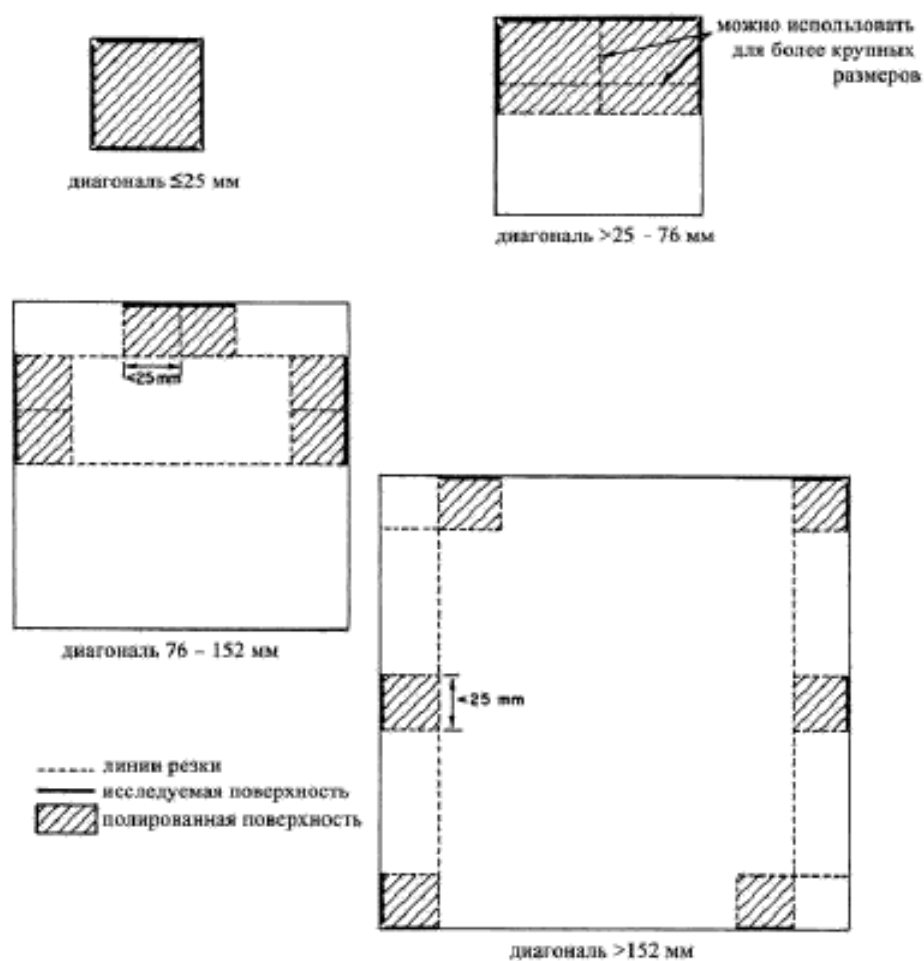
Рисунок 2 – Типичные схемы отбора образцов для квадратных прутков различного размера.
