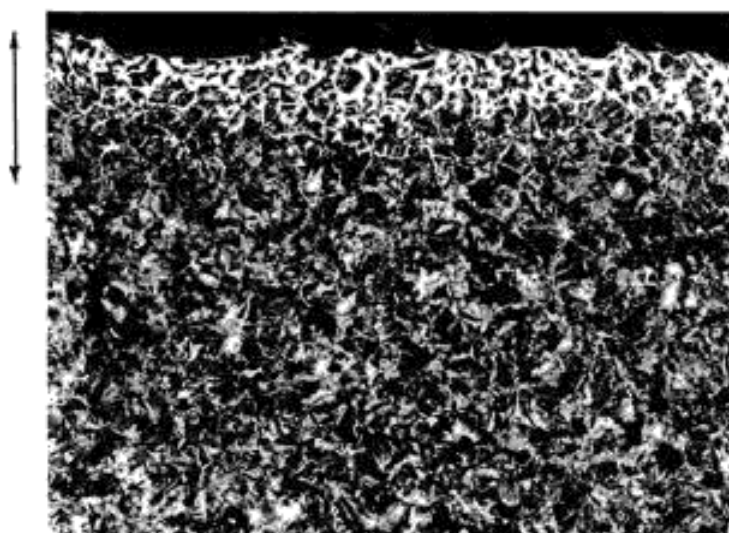
Рисунок 5 – Пример микроструктуры с частичным обезуглероживанием (у поверхности и вблизи нее наблюдается феррит) в полностью перлитной легированной стали в состоянии после прокатки (200×, травление 2 %-ным спиртовым раствором азотной кислоты)
