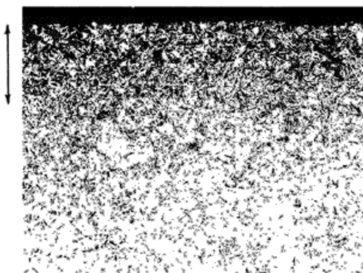
Рисунок 7- Пример частичного обезуглероживания у поверхности образца термообработанной легированной стали с мартенситной структурой (200×, травление 2 %-ным спиртовым раствором азотной кислоты)
