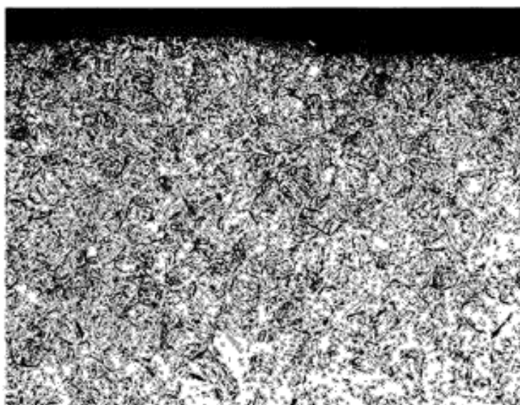
Рисунок 6- Пример микроструктуры (полностью мартенситной) термообработанной легированной стали, в которой не наблюдаются видимые признаки обезуглероживания (200× , травление 2 %-ным спиртовым раствором азотной кислоты)
