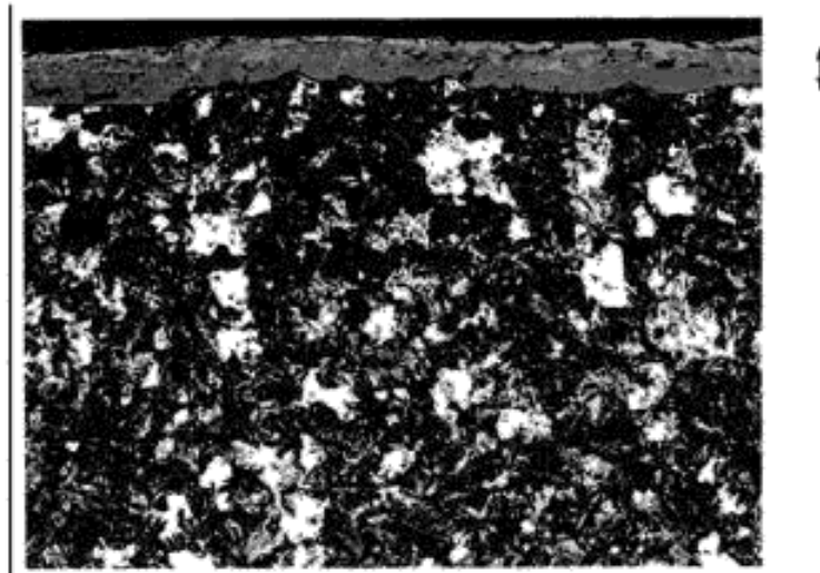
Рисунок 4 – Пример микроструктуры полностью перлитной легированной стали в состоянии после прокатки, в которой не наблюдаются видимые признаки обезуглероживания. Темный слой на поверхности является оксидом железа (прокатной окалиной) (200×, травление 2 %-ным спиртовым раствором азотной кислоты)
