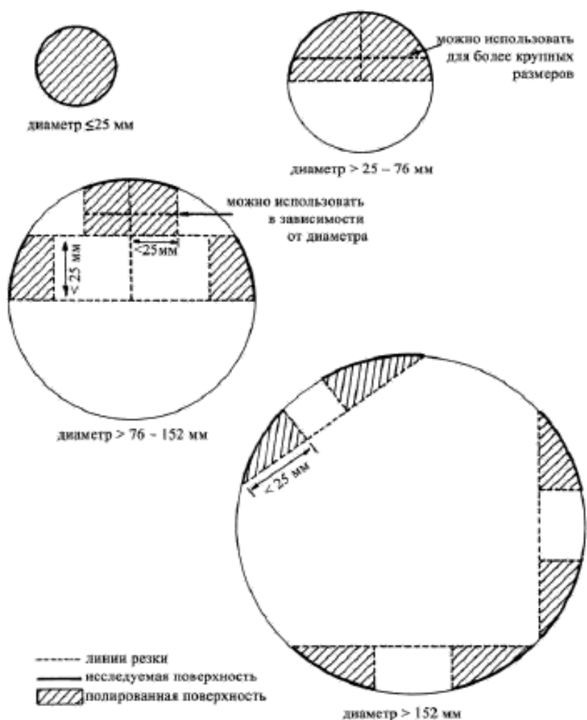
Рисунок 1 – Типичные схемы отбора образцов для круглых прутков различного размера.
