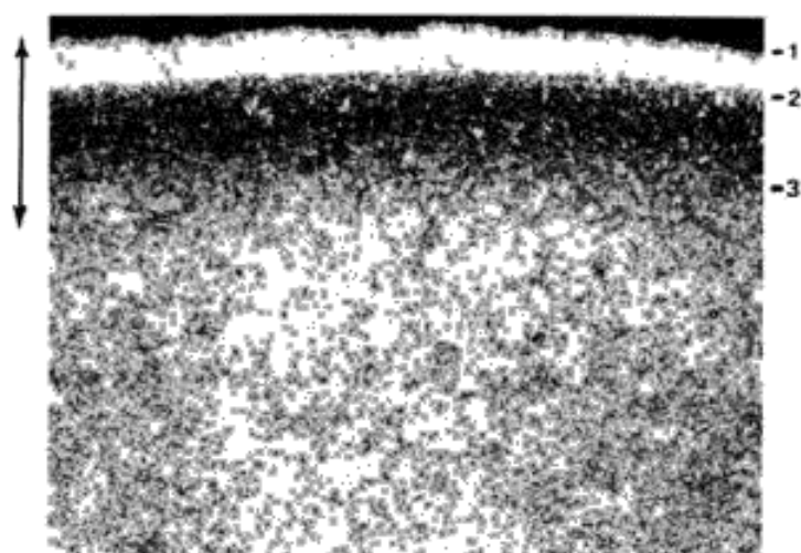
Рисунок 8 – Пример полного обезуглероживания (зона чистого феррита 1 – 2) и частичного обезуглероживания (темная зона 2-3) в термообработанной легированной стали с мартенситной структурой. Общая глубина обезуглероживания равна сумме глубин зон полного и частичного обезуглероживания (1-3) (200×, травление 2 %-ным спиртовым раствором азотной кислоты)
