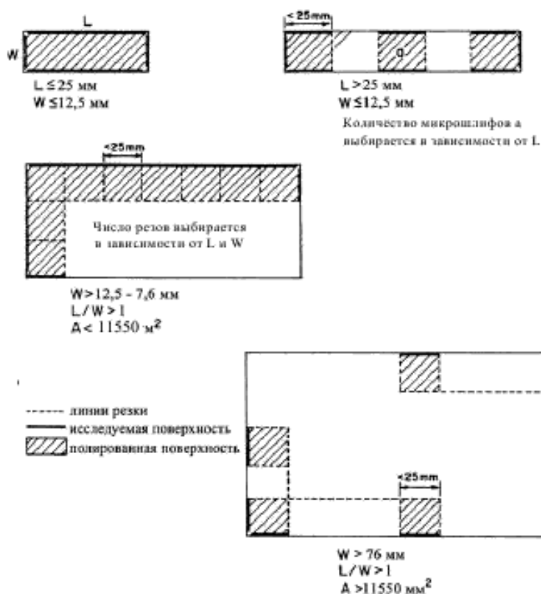
Рисунок 3 – Типичные схемы отбора образцов для плоских и прямоугольных заготовок различного размера.
