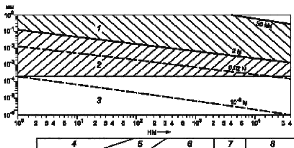
Рисунок А.2 — Соотношение между твердостью по шкалам Мартенса, глубиной индентирования и испытательной нагрузкой
