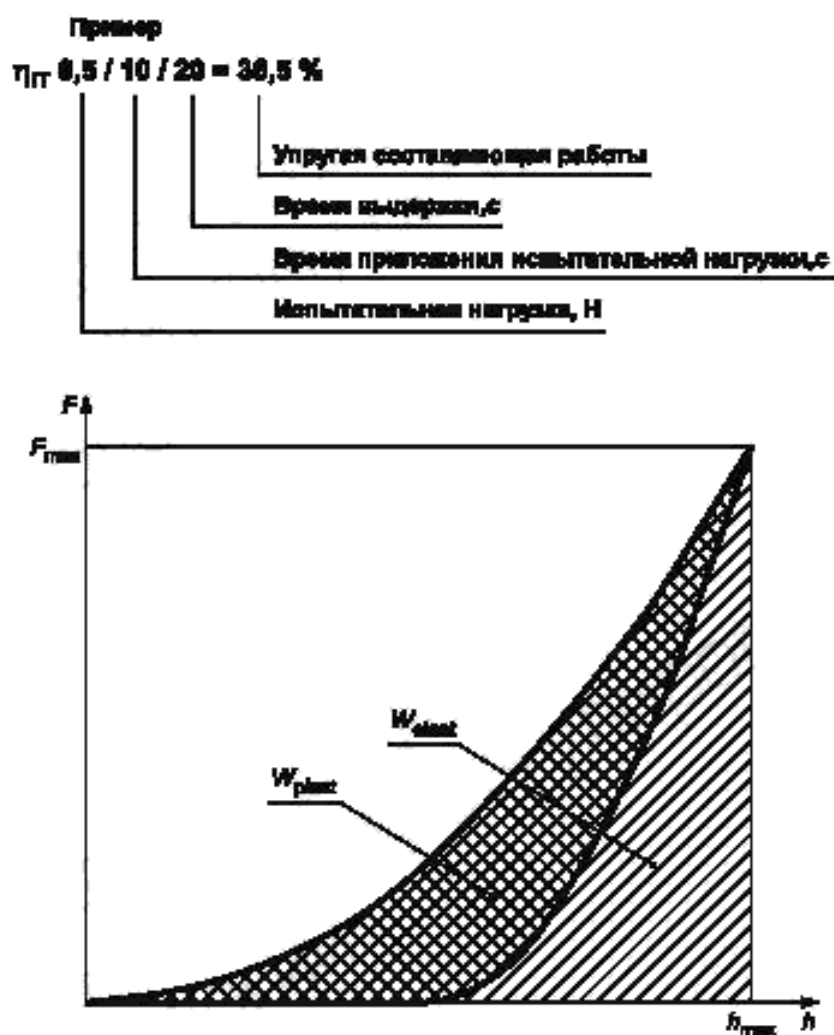
Рисунок А.5 — Пластическая и упругая составляющие работы по индентированию
