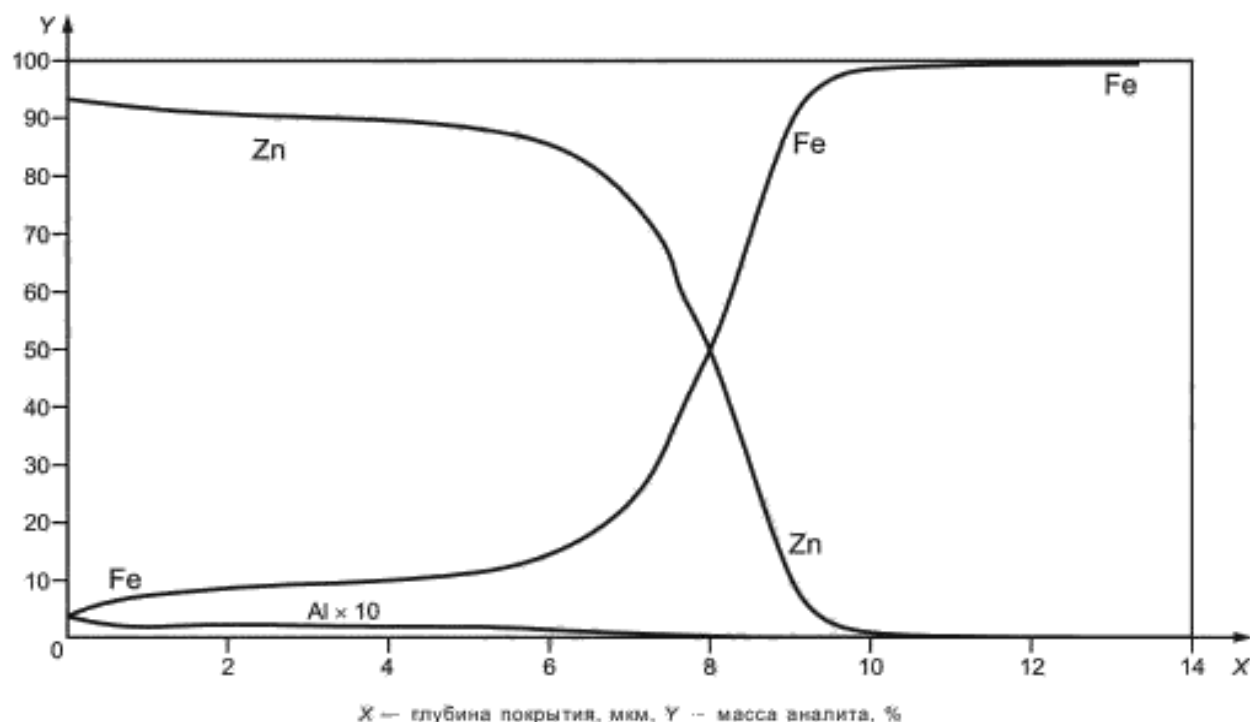
Рисунок 1 — Распределение анализата по глубине гальванического (Zn-Fe) покрытия на стали
