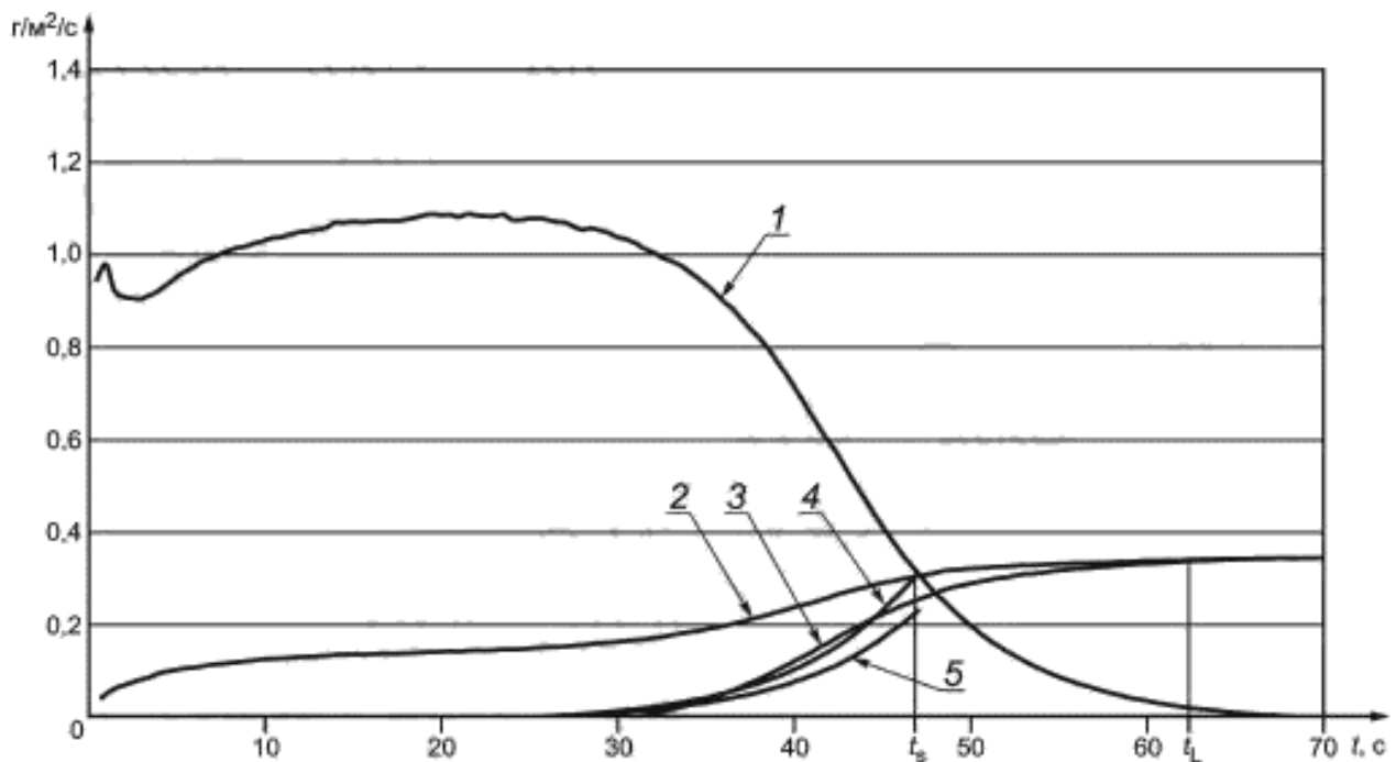
1 — Zn; 2 — Fe; 3 — Fe минус Fe в покрытии; 4 — линия, симметричная линии Zn; 5 — 0,854 \times симметричную линию Z
