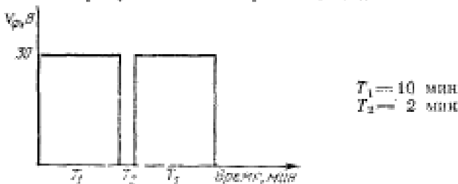
Схема формовки образцов при нормировании на напряжение 30 В
