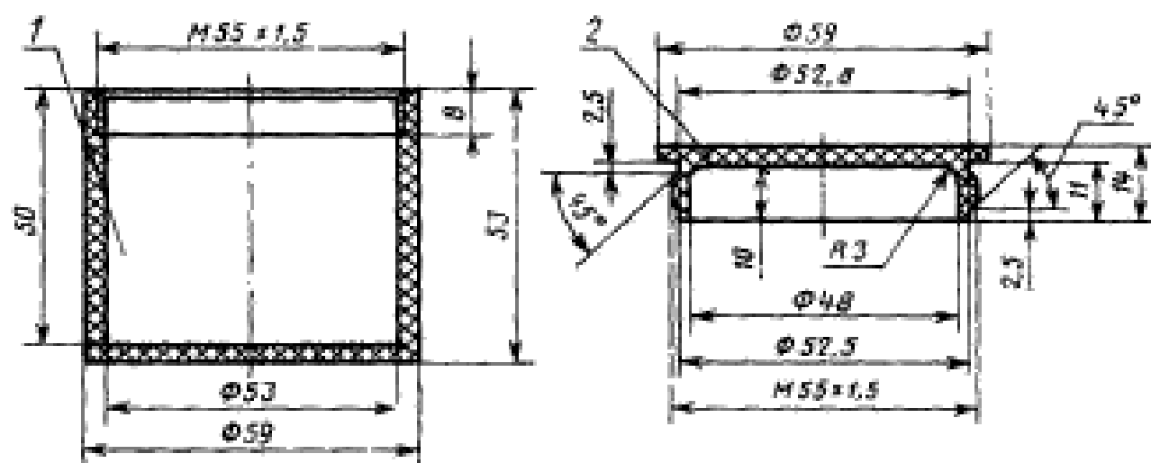
1 — чашка фторопластовая; 2 — навинчивающаяся крышка
