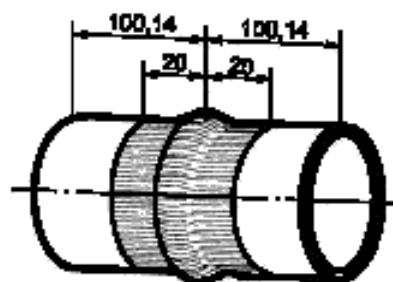
Рисунок Е.2 — Образец для испытаний из трубы, сваренный встык
