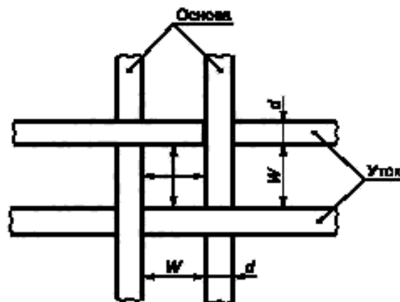
Рисунок 1 — Ячейка сетки
