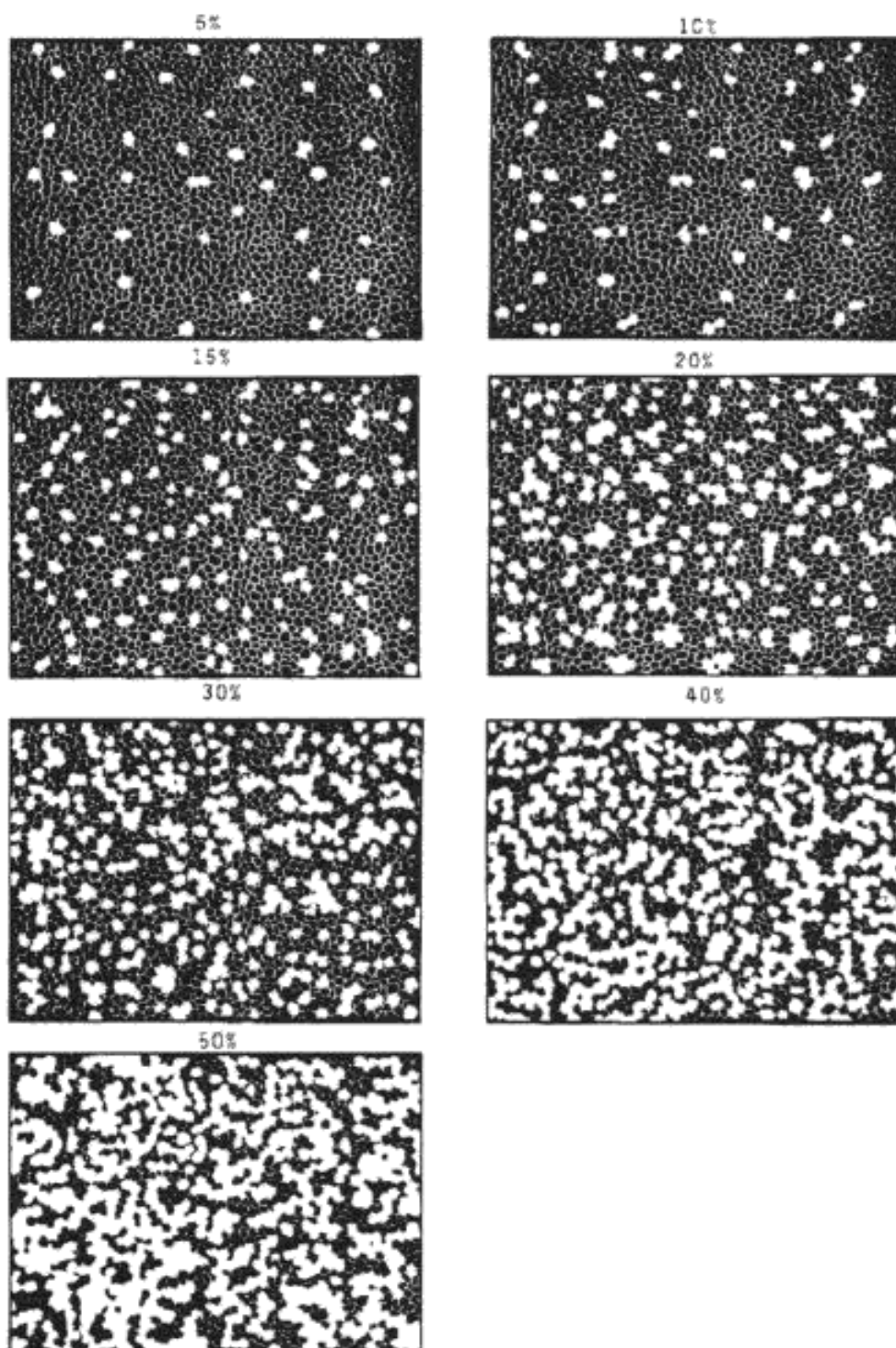
Рисунок А.1 – Эталонная шкала для оценки доли площади, (указана процентная доля площади светлых зерен среди темных зерен)
